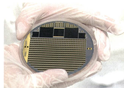
Solarzellenwafer mit Vierfach-Konzentratorsolarzellen und Teststrukturen.
