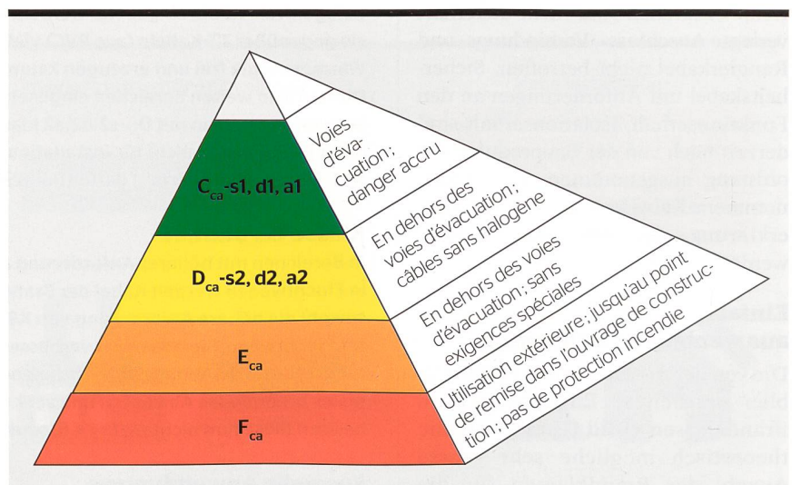
Figure 1 Classes de comportement au feu recommandées par le groupe de travail « CPR-Cable » dans les applications standard.
