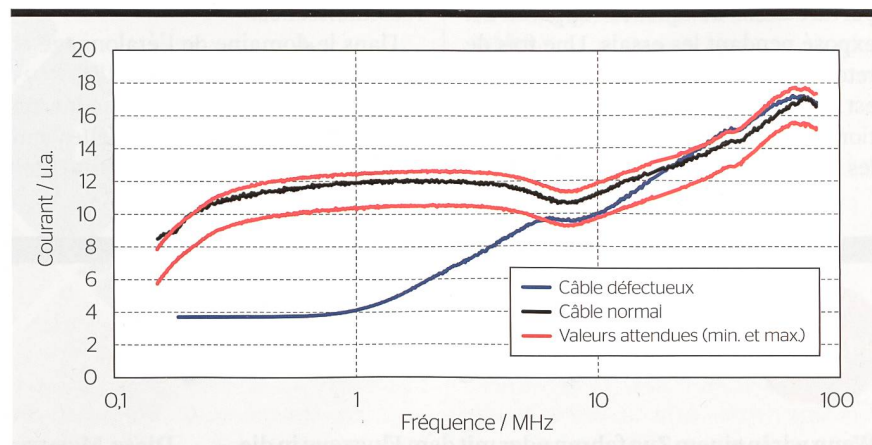
Figure 3 Exemple d'analyse qui permet de démontrer des anomalies dans les montages d'essais. Ci-dessus, le courant mesuré sur le câble d'alimentation en fonction de la fréquence du signal perturbant. Un essai correct devrait fournir des mesures situées entre les deux courbes rouges. Dans le cas de la mesure bleue, un câble présentant un mauvais contact avait été utilisé.
