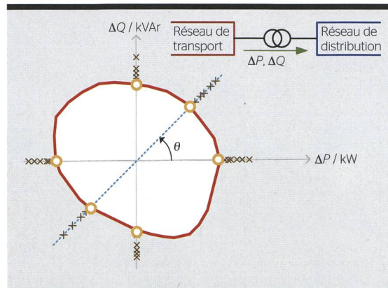
Figure 1 Flexibilité proposée par un réseau de distribution.
