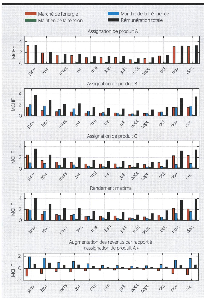
Figure 5 Résultats d'assignations de produit en tenant compte des trois paramètres suivants : réglage secondaire, prix du marché Swissix et priorisation des sources de production décentralisée.
