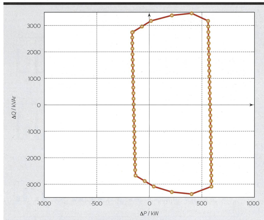
Figure 3 Flexibilité proposée par le réseau d'Aigle (26 juin 2018, à 11h00).
