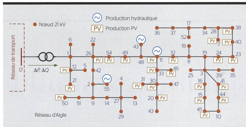
Figure 2 Schéma électrique du réseau d'Aigle.
