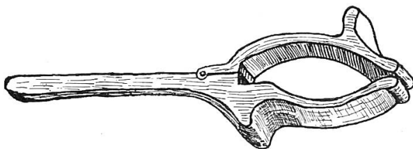
Etau de sellier ou de bourrelier (Etau de selliø ou de bouérreliø)
