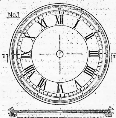
Coupe II-II
