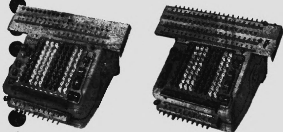
Einzelwerk Rechen-Automat
