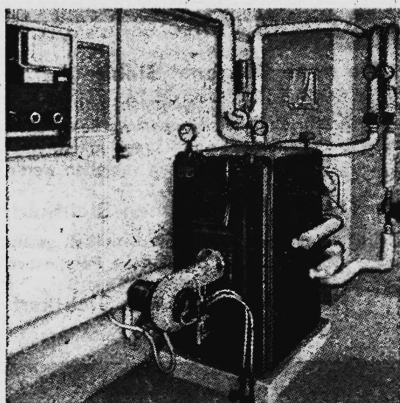
OERTLI-Kleinautomat-Oelfeuerungsanlage im Einfamilienhaus, raum- und boilerthermostatisch gesteuert.
