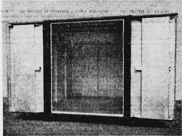
Innenansicht unserer C. T. I. Container Innenmasse: 2,26 × 1,985 × 1,785 m = 8,01 m³
