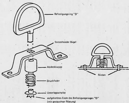
Beispiel eines drehbaren Befestigungsringes (Modell «D»)
