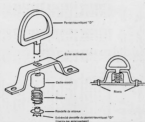
Exemple de pontet-tournequet (modèle «D»)
