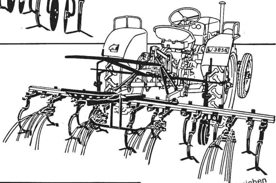
Traktor-Vielfachgerät mit Sitzsteuerung
