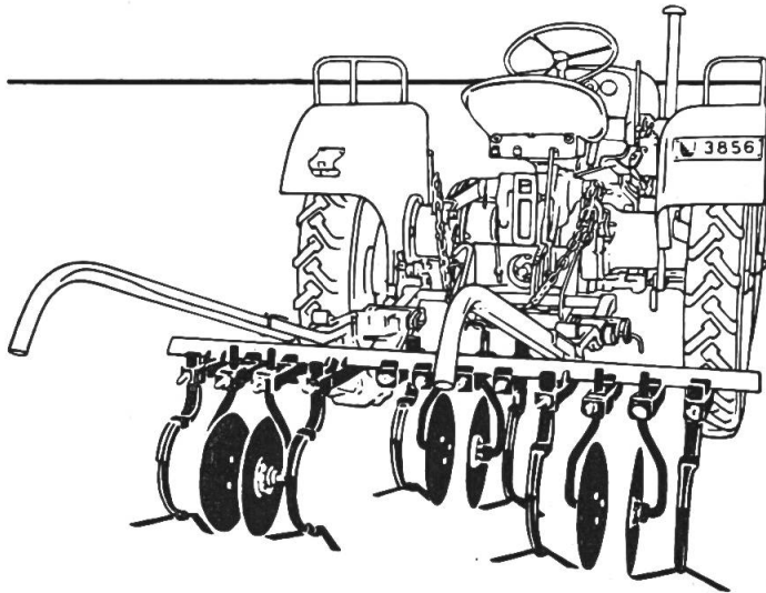
Gespann-Vielfachgerät mit der patentierten Autosteuerung
