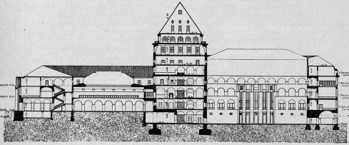
Längenschnitt
