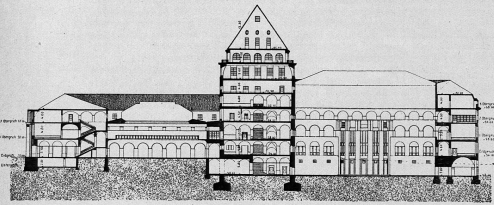
Längenschnitt
