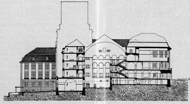
Kollegiengebäude - Querschnitt
