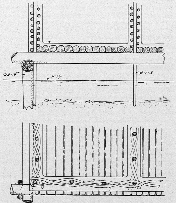
Rost-Konstruktion, schemat. M. = 1:20.
