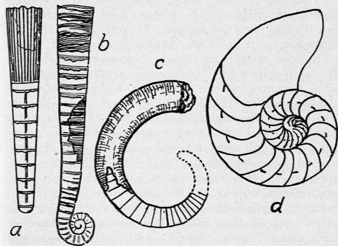
Fig. 2. Nautiloiden oder perlbootartige Kopffüssler. a Orthoceras ; b Lituites ; c Gyroceras ; d Gehäuse des heute noch lebenden Perlboots ( Nautilus ); a bis c nach Fraas; d nach Landois.
