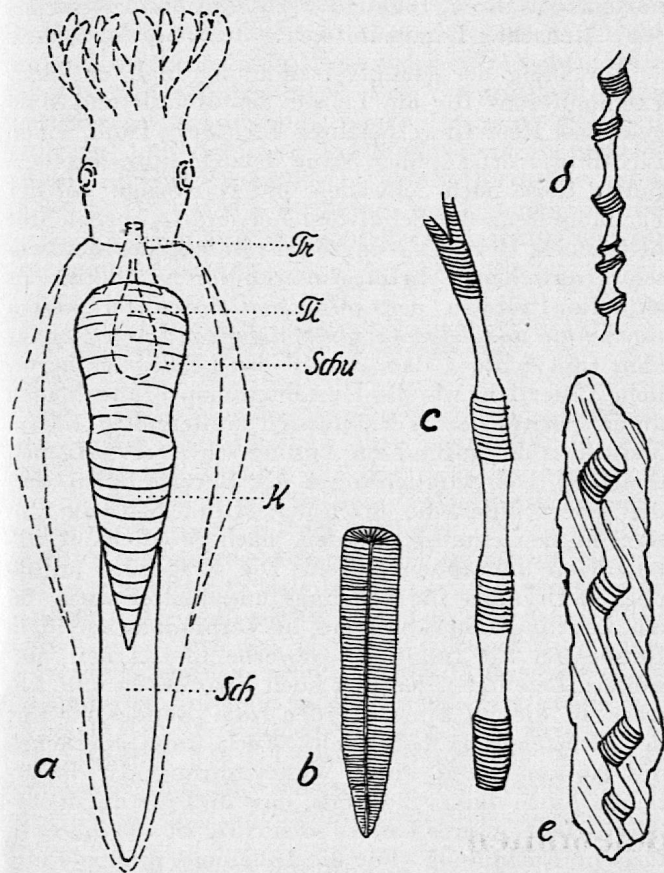
Fig. 1. Belemniten. a = rekonstruiertes Tier, halbschematisch; Tr = Trichter, Ti = Tintenbeutel, Schu = Schulp, K = Kegel, Sch = Scheide; b Hauptteil der Scheide im Längsschnitt; c bis e Deformationen; d und e nach Alb. Heim.
