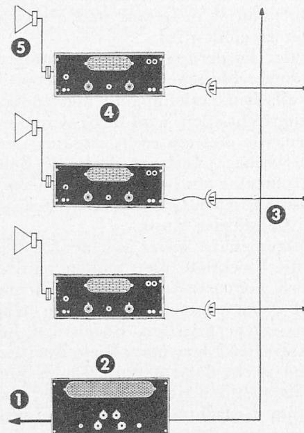
1. Anschluss Telephonrundspruch — 2. Vorverstärker — 3. Leitungsnetz — 4. Kleinverstärker — 5. Lautsprecher
