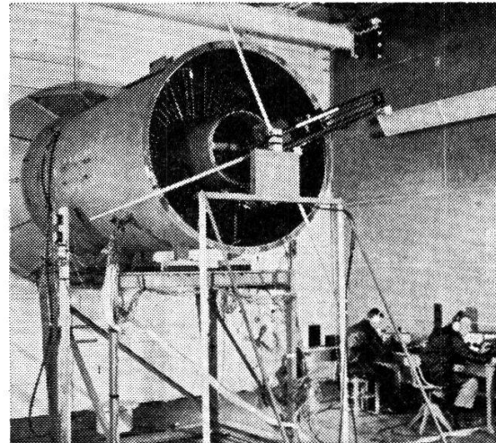
Versuchseinrichtung im Windkanal zur Erforschung Schwingungsverhaltens von Helix-Rohrbündeln Sulzer-Dampferzeuger zu Hochtemperaturreaktoren.
