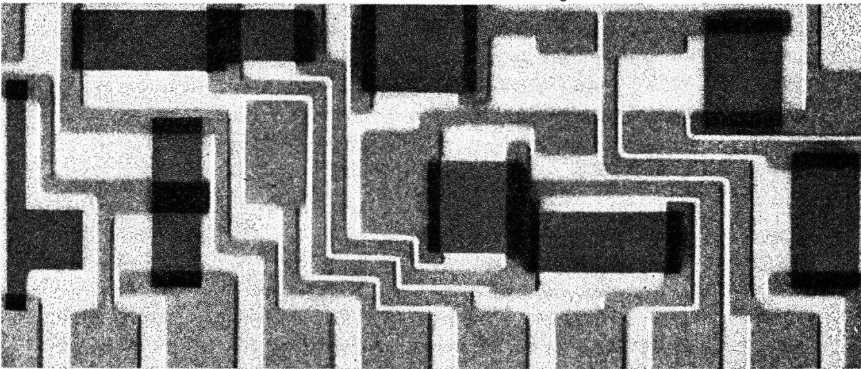
Dickfilmschaltung / Ausschnitt
