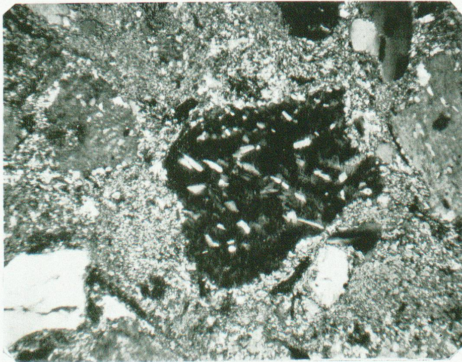
Photo n° 4. Pâte quartzo-feldspathique séricitique cimentant des fragments de quartz et de feldspath potassique à inclusions microlitiques d'albite. Echantillon Roffna n° 2. G = 20 ×. Nicols croisés.
