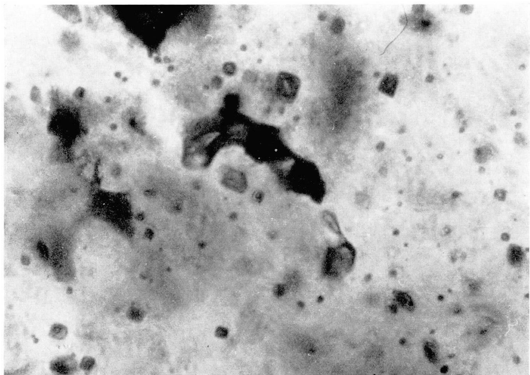
Fig. 2. Remplissage d'une cavité (en forme de bâtonnet) par plusieurs particules d'or (parties sombres) et par la phase fluide constituée par H_2O . \times 600 .
