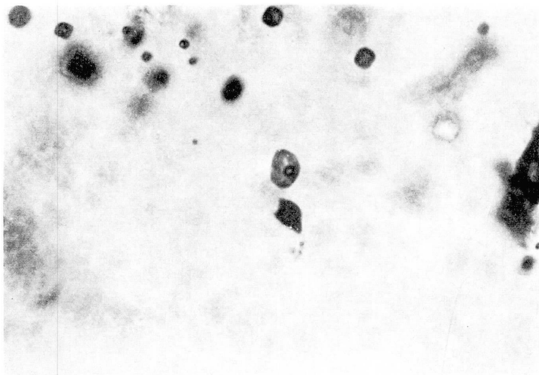
Fig. 3. Particule d'or (partie sombre) au voisinage d'une cavité remplie de H 2 O et CO 2 . × 400.
