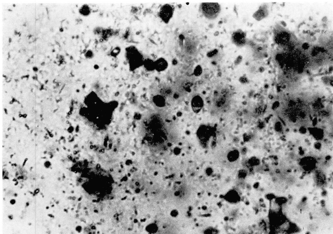
Fig. 4. L'association d'ensemble de nombreuses inclusions fluides monophasées et diphasées et de particules d'or (parties sombres et localement semi-transparentes). × 400.
