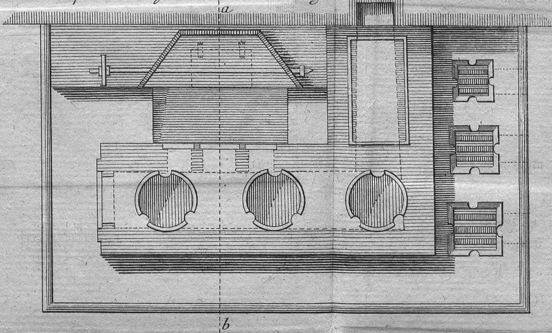
Coupe du Foyer oultre sur la ligne a. b.
