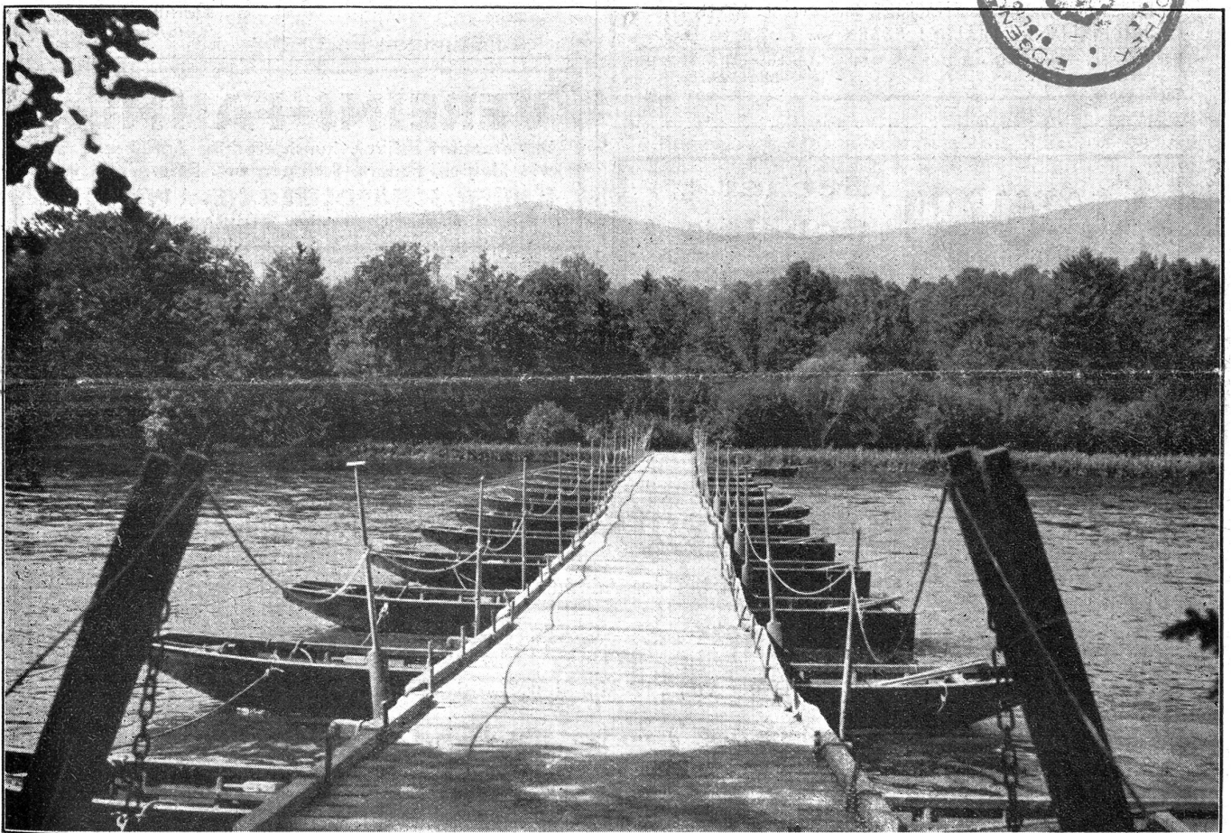
Pontonbrücke mit Flussverankerung — Pont de pontons avec ancrage.
