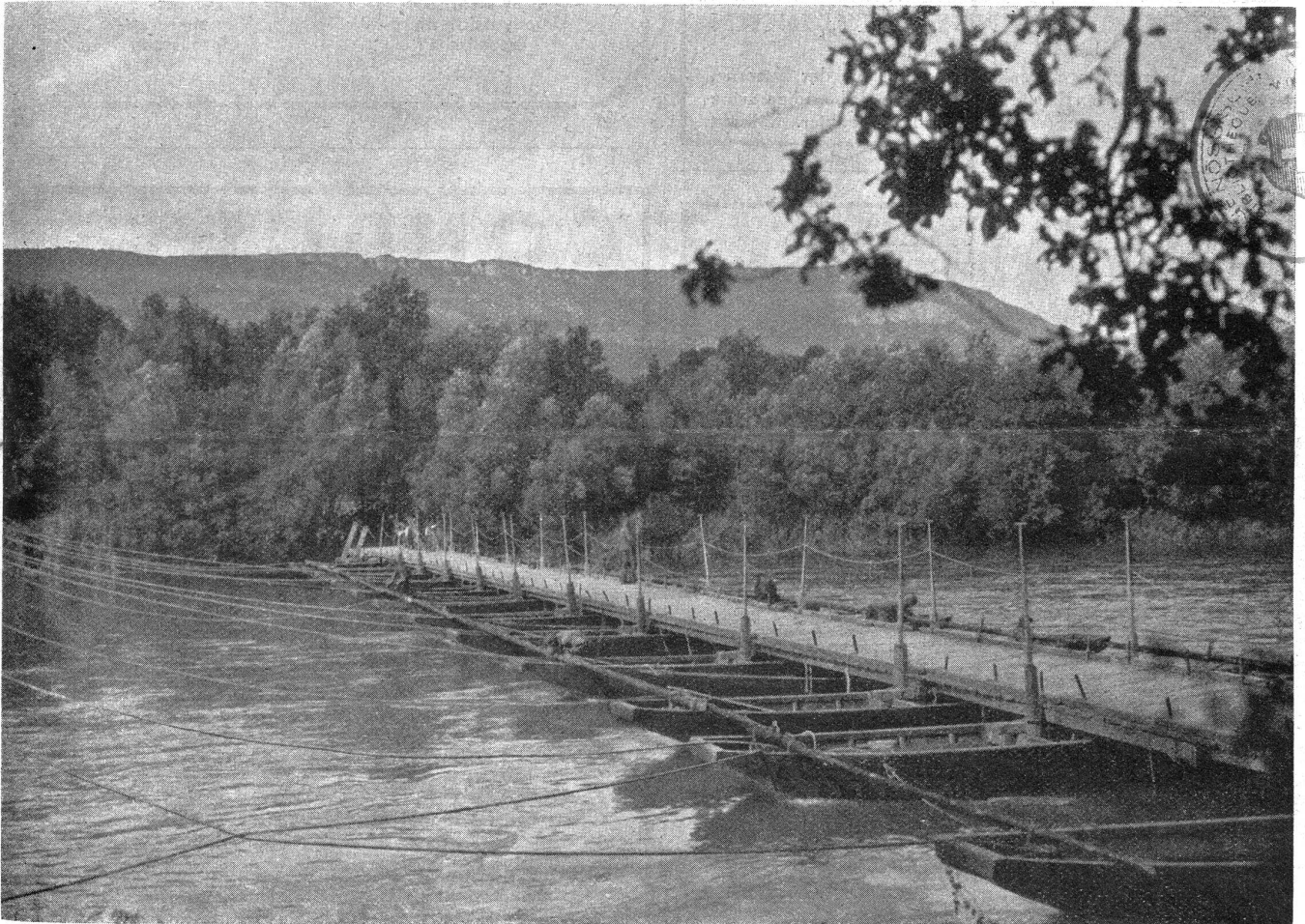
Schertaubücke. — Die Pontons hängen an einem über den Fluss gespannten Drahtseil, dem sogen. Schertau. Pont à cinquenelle. — Les pontons sont accrochés à un câble dit cinquenelle tendu sur la rivière.
