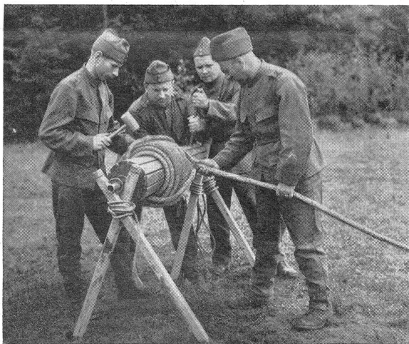
Rollen eines Schlepptaues. Enroulement d'une corde traînante.
