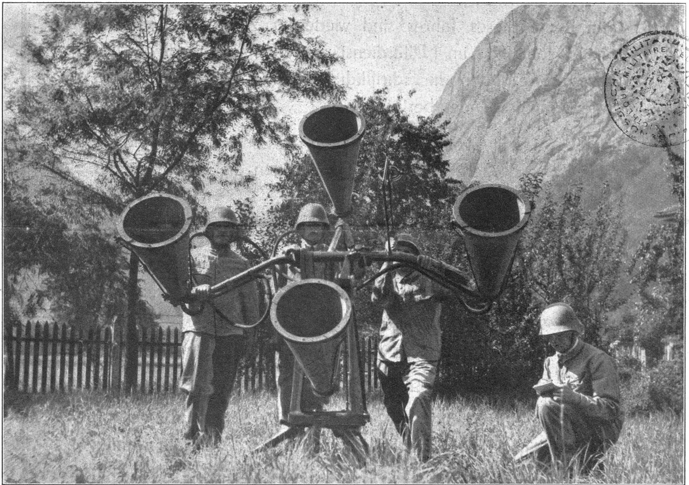
Passiver Luftschutz. — Horchgerät eines schweizerischen Fliegerbeobachtungspostens mit Bedienungsmannschaft Phot. K. Egli, Zürich Protection passive contre les gaz. — Appareil d'écoute d'un poste suisse d'observation aérienne avec équipe de servants
