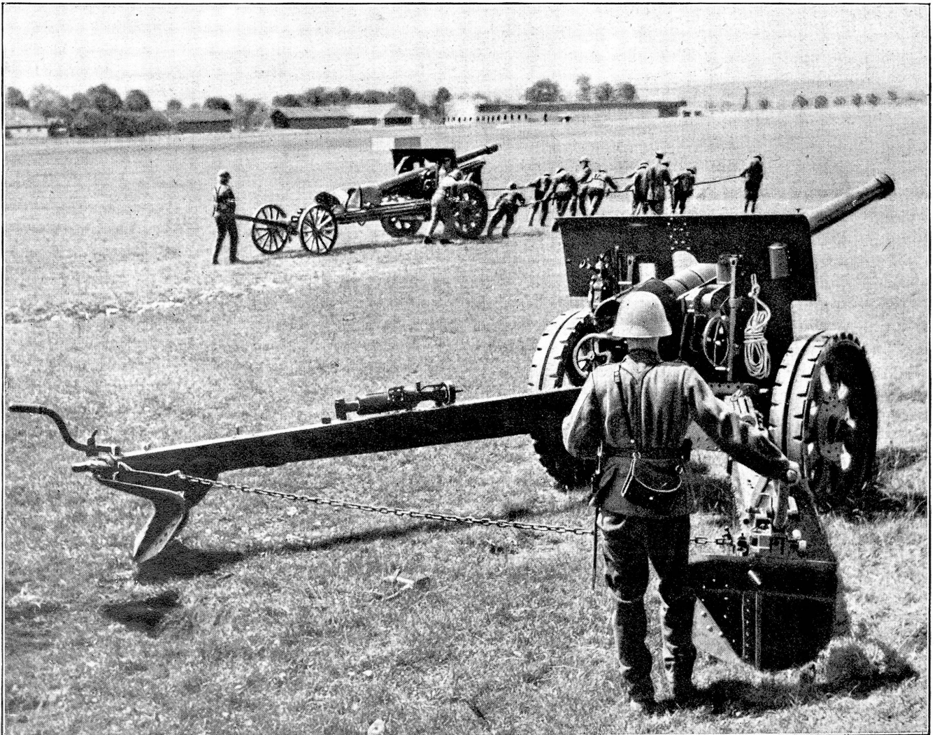
Unser neuestes Geschütz. Die Oefnung der beiden Spreizen beträgt etwas über 4 m. Durch diese Lafettenkonstruktion wird eine stärkere Standsicherheit des Geschützes durch Teilung der Rückstoßwirkung des Schusses erreicht. Im Mittelgrund wird eben das zweite Geschütz eines Zuges von den Bedienungsmannschaften in Stellung gebracht.
