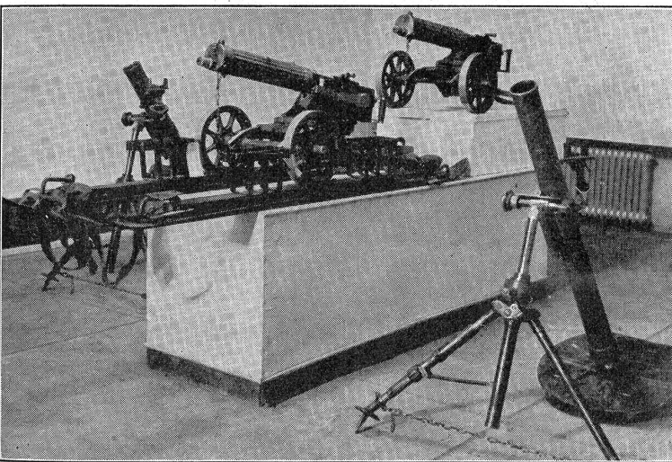
Rechts: Bild Nr. 2: 8,1-cm-Minenwerfer, System Stockes-Brandt, der in Bau und Leistungen dem schweizerischen Mw. entspricht. — Mitte: 7,62 mm schwere Mg., System Maxim Mod. 1910, auf Räderlafette, die 41 kg wiegt. Unteres Mg. zudem auf Skikufen montiert.
