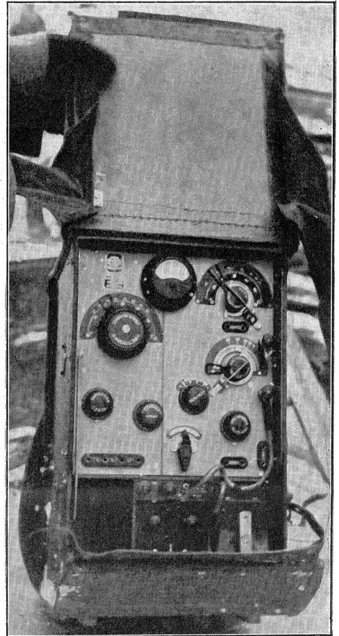
Bild Nr. 3. Russische T.L.-Funkstation. Station radiotélégraphique. Stazione radio russa.
