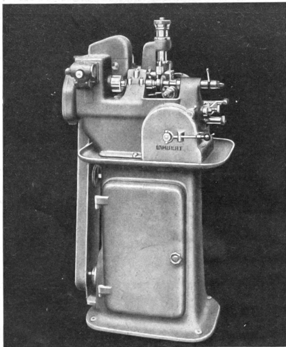
Abwälräderfräsmaschine Type 75
