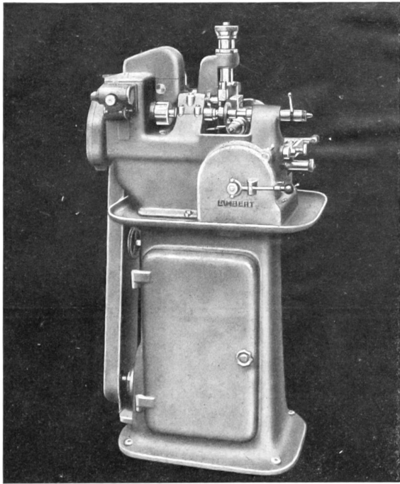
Abwälzräderfräsmaschine Type 75
