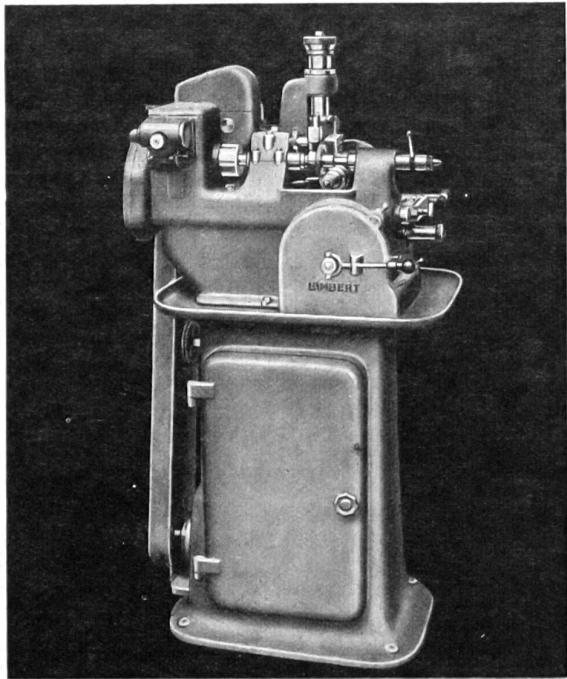
Abwälzräderfräsmaschine Type 75
