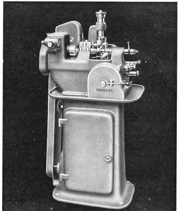
Abwälzräderfräsmaschine Type 75
