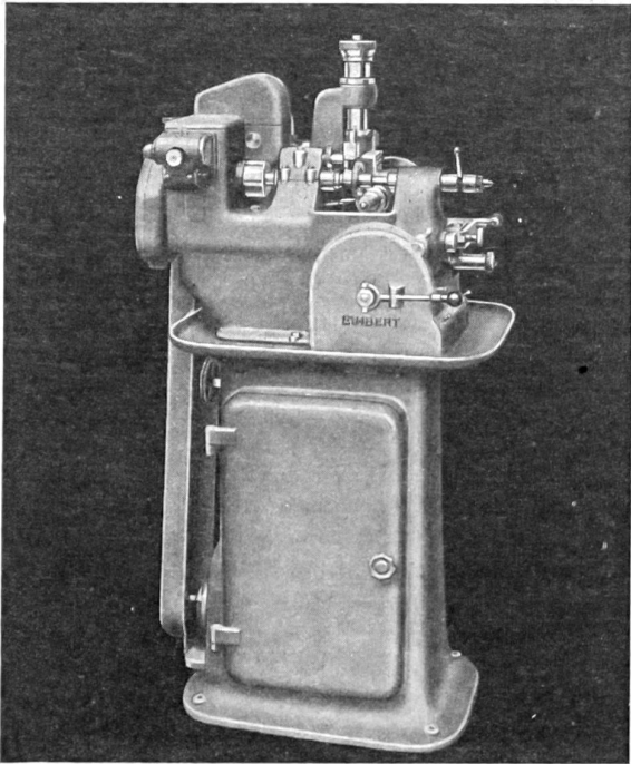
Abwälzräderfräsmaschine Type 75
