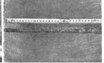
Wirkung der Hohlladung 8-cm-Panzerrakete
