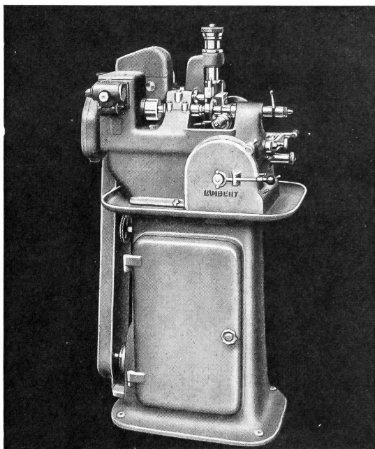
Abwälzräderfräsmaschine Type 75
