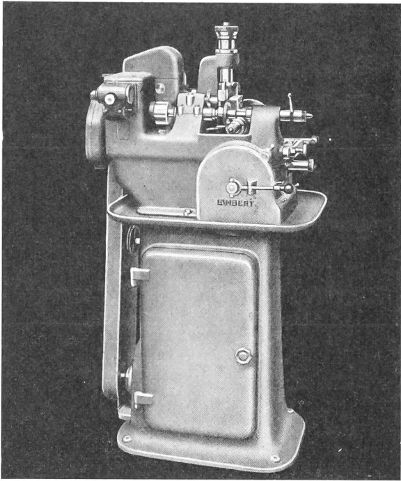
Abwälzräderfräsmaschine Type 75
