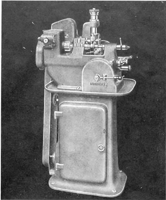
Abwälzräderfräsmaschine Type 75
