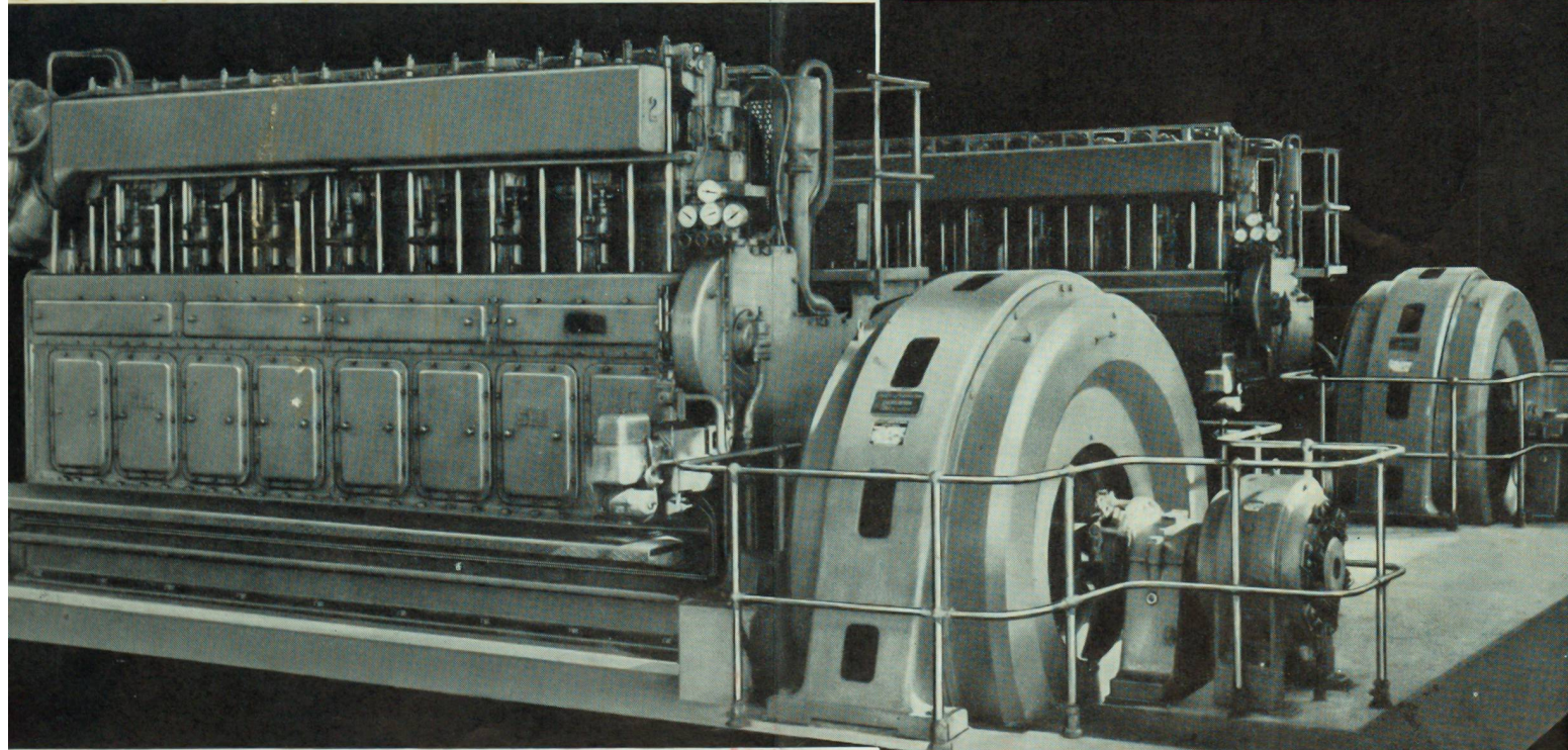
— Dieselmotorenanlage in Libanon, Leistung 2 x 1200 PS bei 500 U/min —
