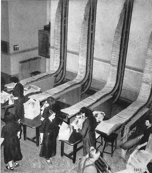
Zeitungsförderanlagen
