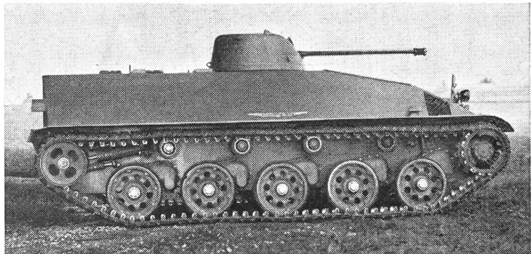
Schützenpanzerwagen Pirat ▶
