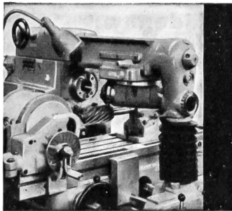
Maschine ausgerüstet mit Universal-Teilapparat
