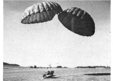
1 Der Abwurf des Kleinfahrzeuges A.S. 24, das nur 220 kg wiegt, erfolgt an zwei normalen Fallschirmen. Es kann von zwei Mann innert einer Minute einsatzbereit gemacht werden.
