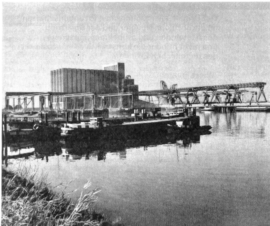
BÜHLER-Umschlags- und Siloanlage im Hafen Botlek (Rotterdam) Leistungen: Entladung = 1600 Tonnen pro Stunde, Beladung = 2800 Tonnen pro Stunde!
