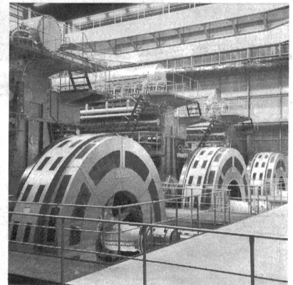
Afrikas grösstes Dieselelektrizitätswerk «Bong Range» in Liberia wird im Endausbau rund 100000 PS Gesamtleistung haben. Die auf dem Bilde gezeigten Sulzermotoren vom Typ 9RF68 entwickeln je 13500 PS Nennleistung.
