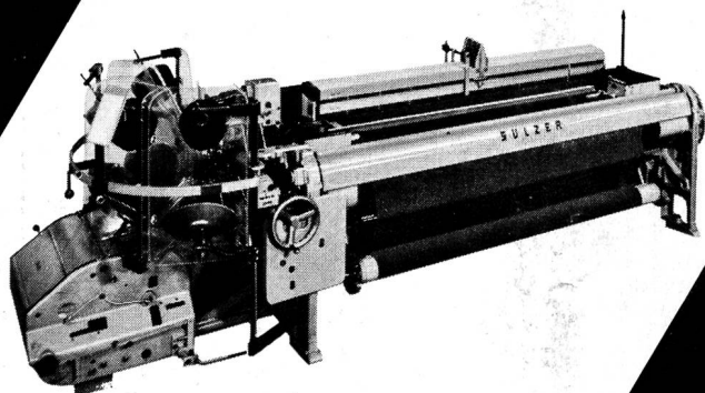
Sulzer-Webmaschine
