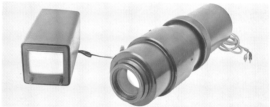
Restlichtverstärker-Kamera (LLL-TV)
