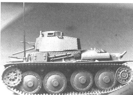
Unterschiede Pz KpW 38 (t) — Pz 39. Bewaffnung: Hauptbewaffnung: Pz 39 mit Mündungsbremse und 24-mm-Kanone sowie Pz Mg 38.
