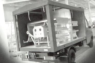
FHS-Spezial-Wechselaufbau
