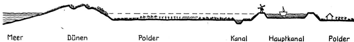
Schnitt durch das Polderland
