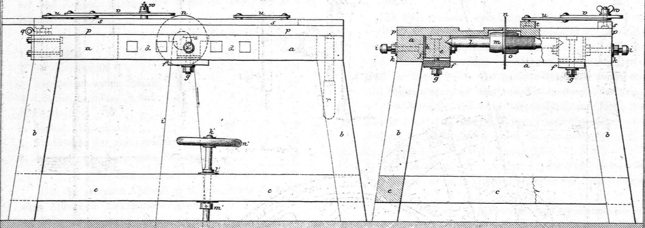
Fig 3. Querschnitt.
