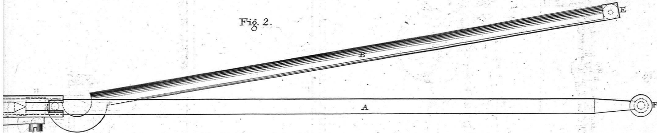
Libellen-Dezimalwaage von Pfanzeder. Maßstab 3/2.
