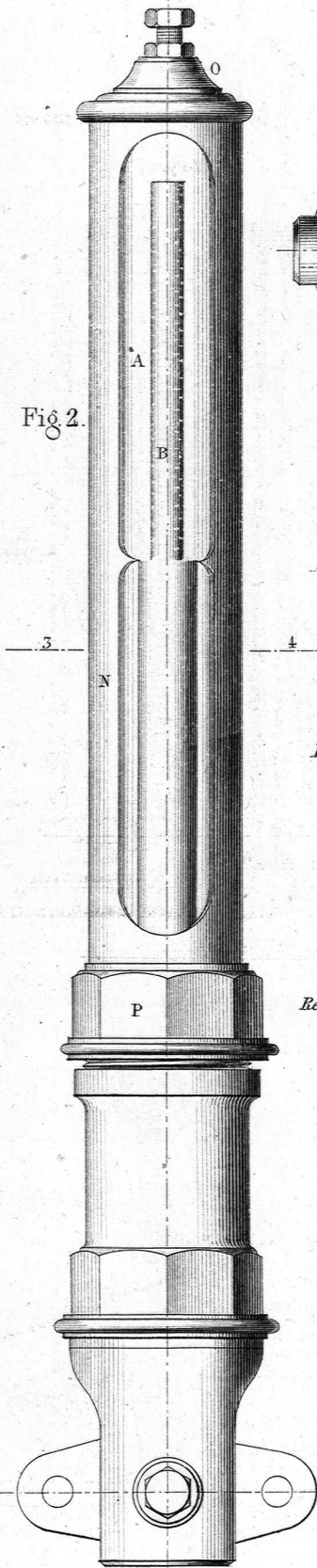
Wasserstandzeiger von F. Reuleaux. Maßstab = 1/2.
