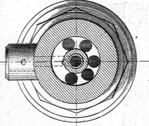
Fig. 3. Schnitt nach 1-2.
